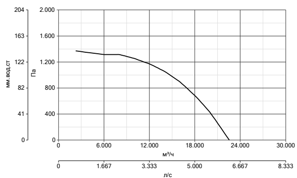
HEATMASTER F400 630 T4/T8 5.5/1.1KW артикул 15310
